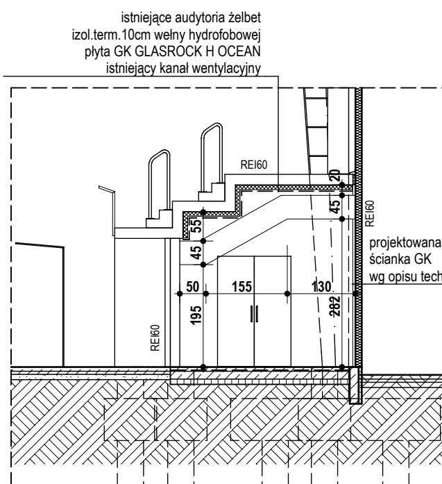
SZKIC ISTNIEJĄCEGO PRZEBIEGU KANAŁÓW WENTYLACYJNYCH W POMIĘSZCZENIACH SZATNI
